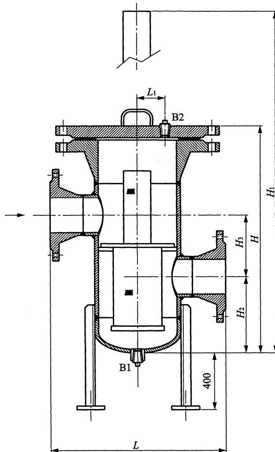
图 5.4.4-1 法兰连接多滤筒式篮式过滤器结构
