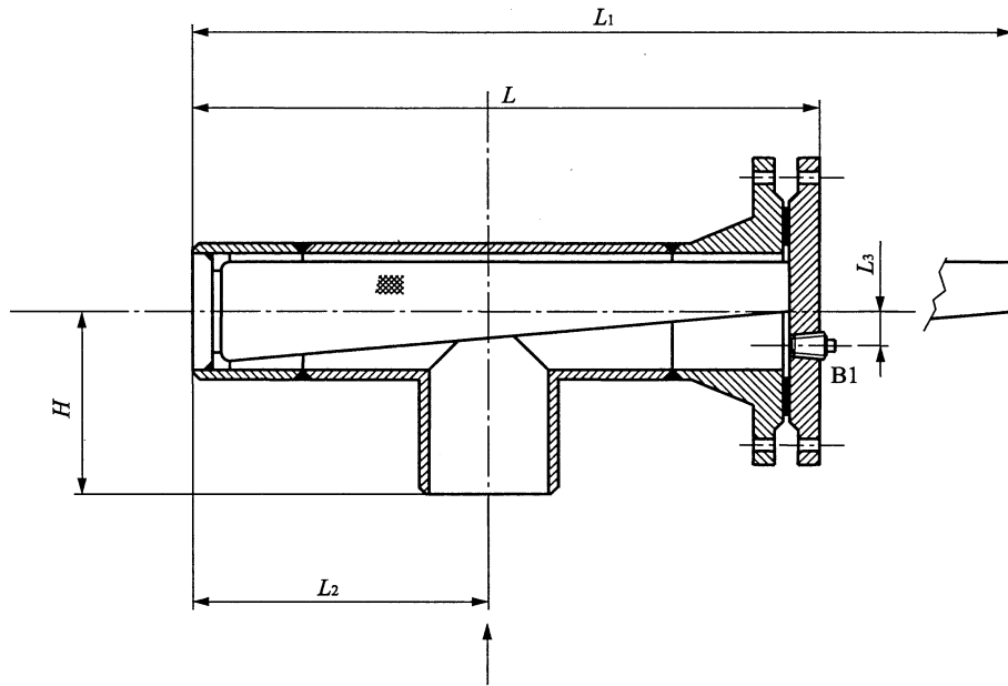
图 5.2.6 反折流式焊接连接 T 形过滤器结构
