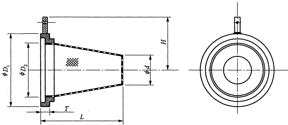
图 5.3.3-2 法兰密封面型式为凹凸面的平顶式锥形过滤器结构
