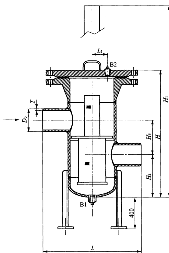
图 5.4.4-2 焊接连接多滤筒式篮式过滤器结构
